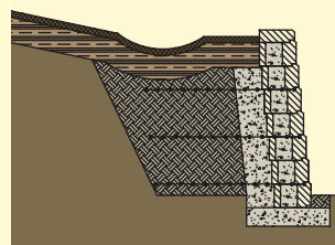
Swales
