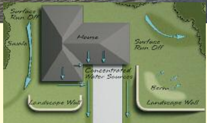
Swales
